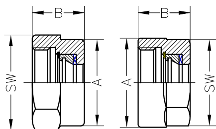
HTG 75
